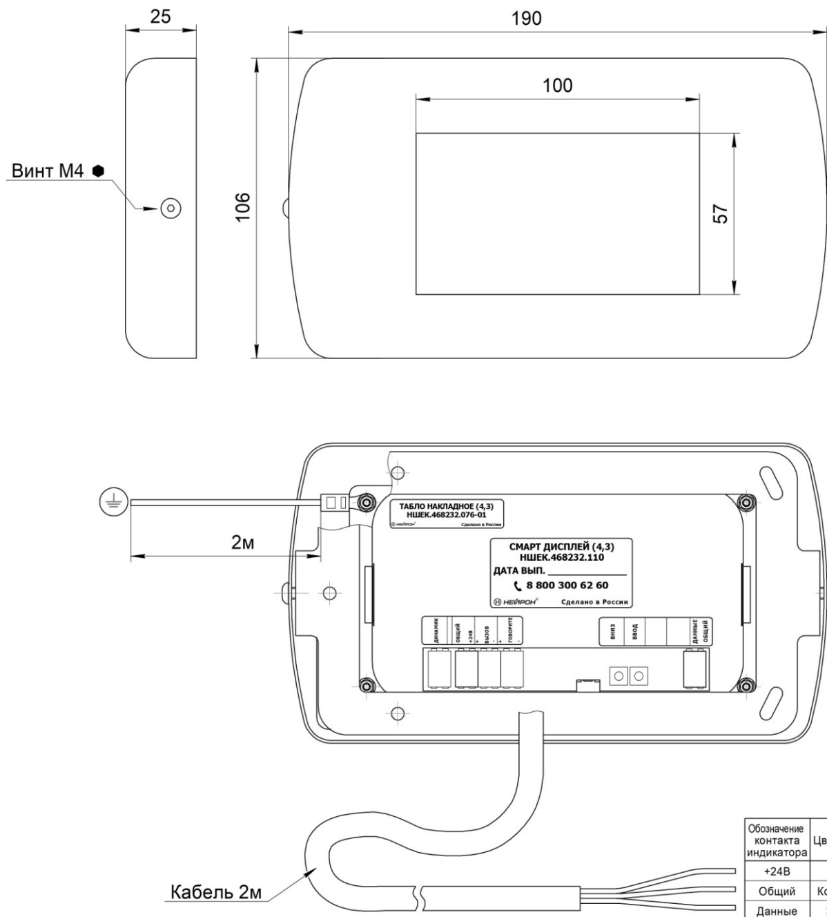
Рис.1 Внешний вид Табло накладное (4,3) НШЕК.468232.076-01
